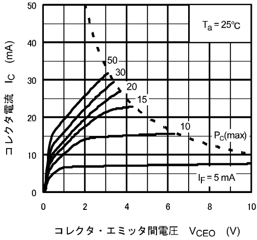
図 11.7 I_C - V_{CE0}
