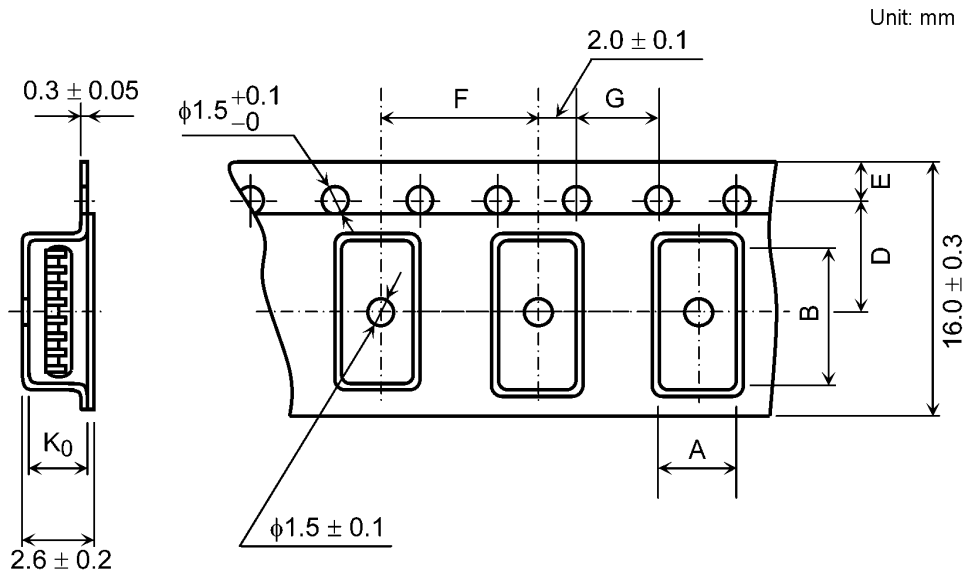
図 15.3.5.1 テープ形状
