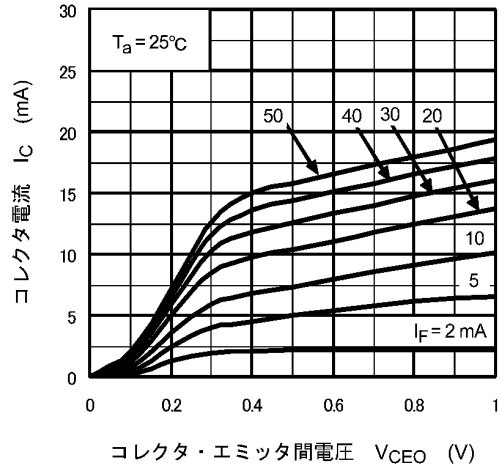
図 11.8 I_C - V_{CE0}
