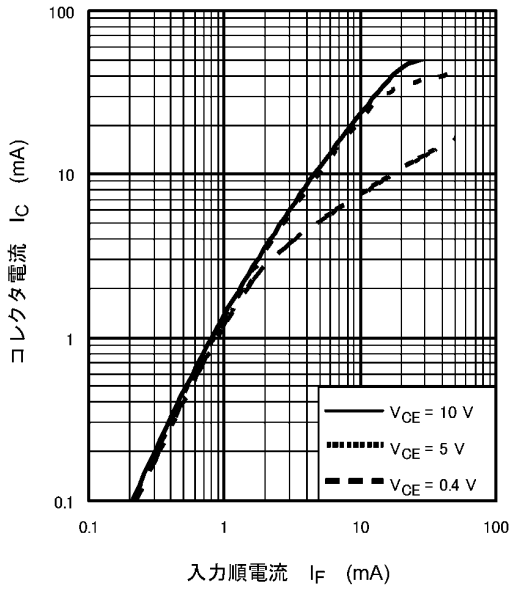
図 11.9 I_C - I_F
