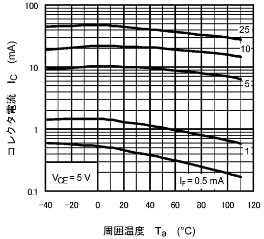
図 11.13 I_C - T_a
